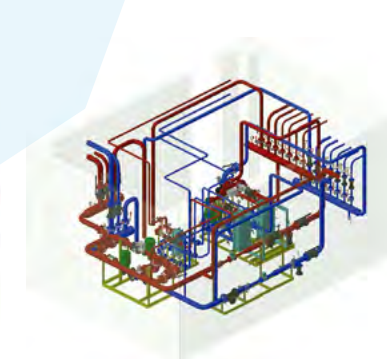
Тепловой пункт здания с узлом учета тепловой энергии и обвязкой модулей отопления и ГВС
