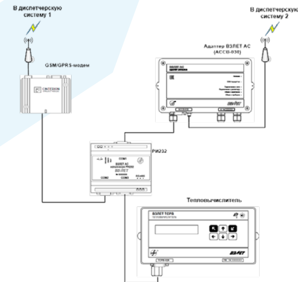
Пример организации информационного обмена одного прибора с двумя диспетчерскими системами с использованием RI232
